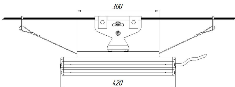
Светильник УСС 90 МАГИСТРАЛЬ Ш с 2Ех маркировкой крепление на трос
