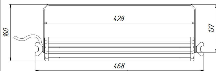
Светильник УСС 90 МАГИСТРАЛЬ Ш с 2Ех маркировкой крепление скоба
