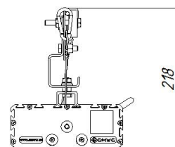
Светильник УСС 90 МАГИСТРАЛЬ Ш с 2Ех маркировкой крепление на трос
