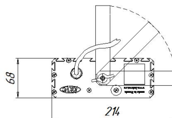
Светильник УСС 90 МАГИСТРАЛЬ Ш с 2Ех маркировкой крепление скоба
