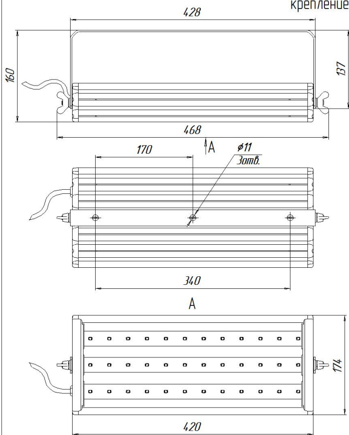
Светильник УСС 36 с 2Ех маркировкой крепление скоба
